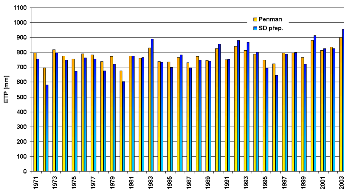
Porovnání ročních hodnot podle Penmana a přepočítaného syt. doplňku pro Hurbanovo
