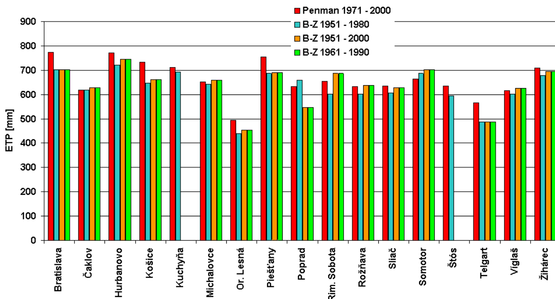
Potenciální evapotranspirace podle Penmana a Budyka se Zubenokovou
