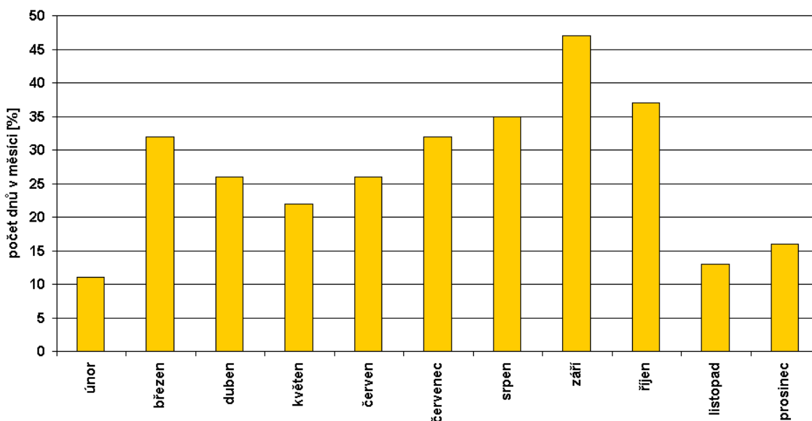
Obr. 10 Relativní četnost dnů s rozdílem minimálních teplot mezi Děvinem a Lednicí větší než 2 °C
