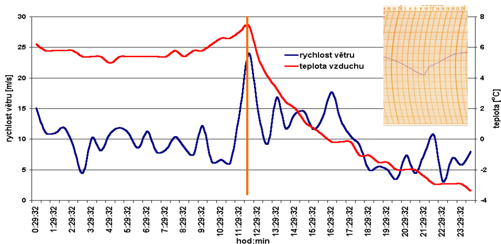
Průběh teploty vzduchu a rychlosti větru dne 19.11.2004
