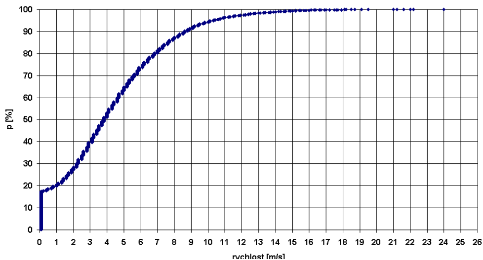
Obr. 4 Čára překročení rychlostí větru v roce 2004
