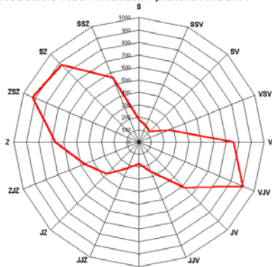
Obr. 6 16-ti dílná větrná růžice pro Děvín za rok 2004
