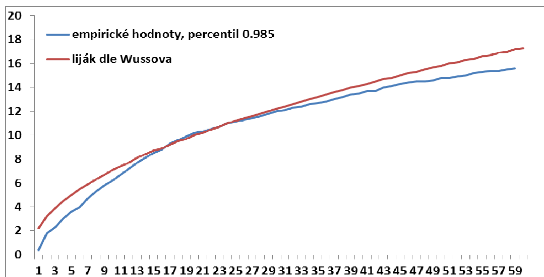
Obr. 6 Porovnání hranice pro liják podle Wussova pro délky trvání deště 1–60 minut s hodnotou extrémního percentilu stanoveného z empirických dat z vybraných stanic na území brněnské pobočky ČHMÚ za období 2009–2013
