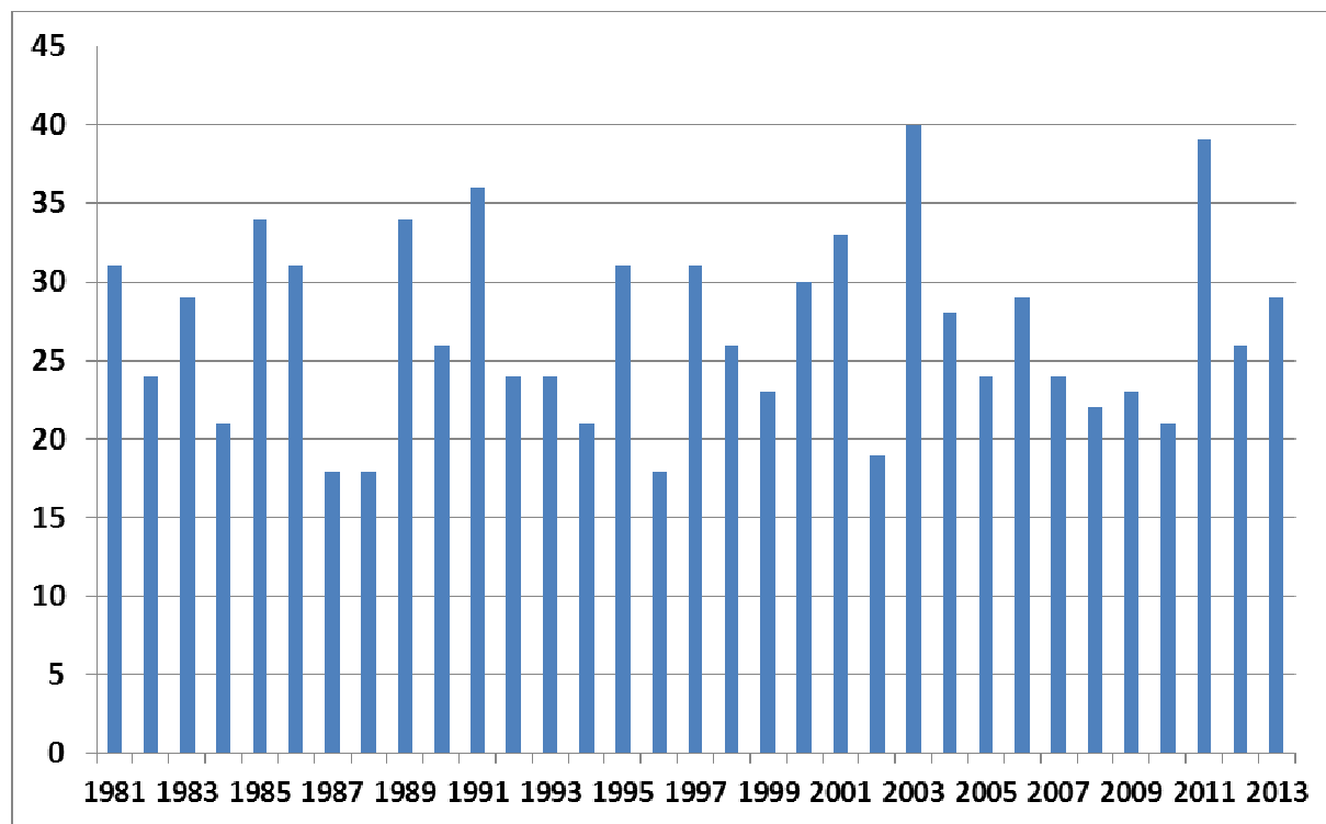
Obr. 2 Maximální délka suché periody (ve dnech) na stanici Kroměříž v období 1981–2013
