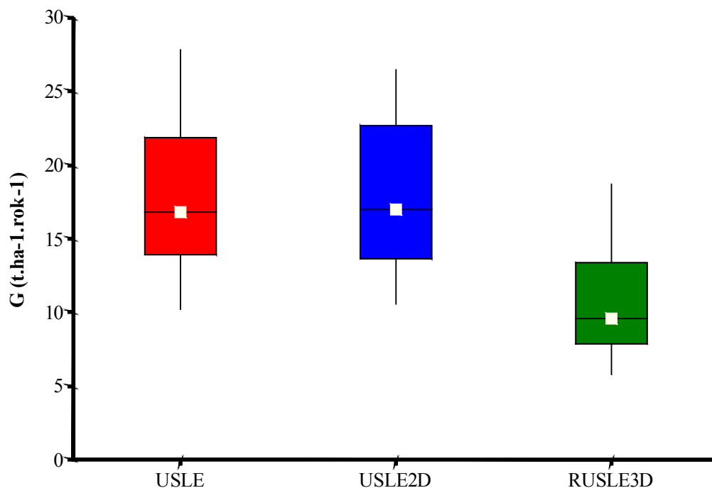
Obr. 7 Krabicový graf s bíle zaznačenými průměry všech hodnot smyvu půdy stanovených na základě modelů USLE, USLE2D a RUSLE3D
